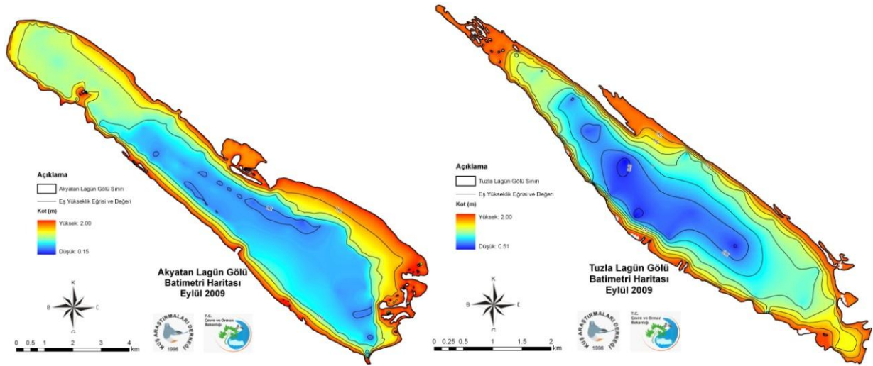
Harita 7: Akyatan ve Tuzla lagünleri derinlik (batimetri) haritaları
